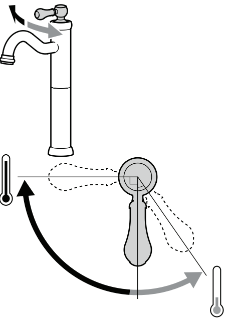
Diagrama, ki prikazuje, kako se s pomočjo ročice odpreta hladna in topla voda.
